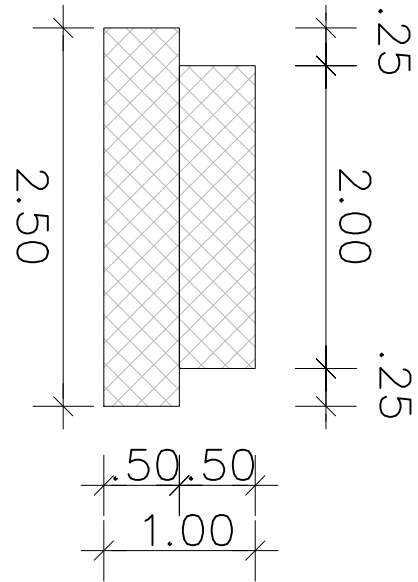
Prerez 2 - 2:
